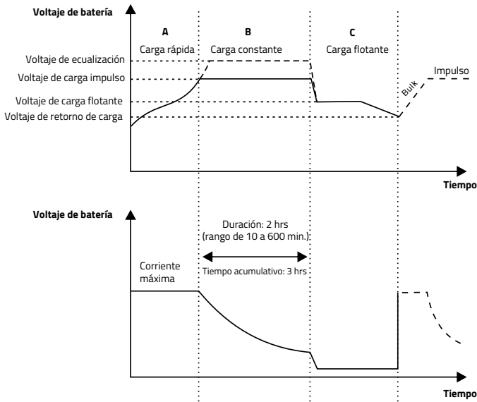
Diagrama de las etapas de carga de la batería
