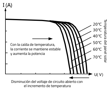
Fig. 1-3 Relación entre las características de salida del panel solar y la temperatura
