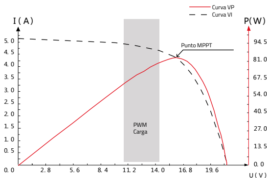
Fig. 1-2 Curva característica de potencia de salida de un panel solar (ejemplo de un panel utilizado en sistemas de 12 Vcd)
