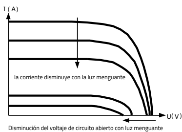
Fig. 1-3 Relación entre las características de salida del panel solar y la iluminación
